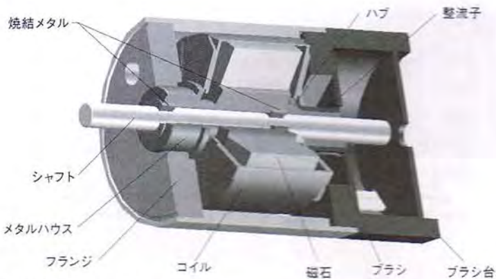
図7●開発したコアレスモータの構造図 コイルが磁石を包囲している。まるで鳥かごのよう。一体、どうやって通るのだろうか。
